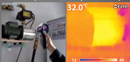
La thermographie permet d'identifier rapidement les problèmes électriques et mécaniques.
