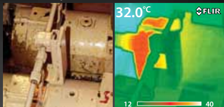
Vérification mécanique d'un moteur électrique avec la FLIR Série i.
