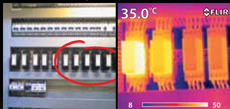
Inspection d'un fusible défectueux avec une caméra thermique FLIR.
